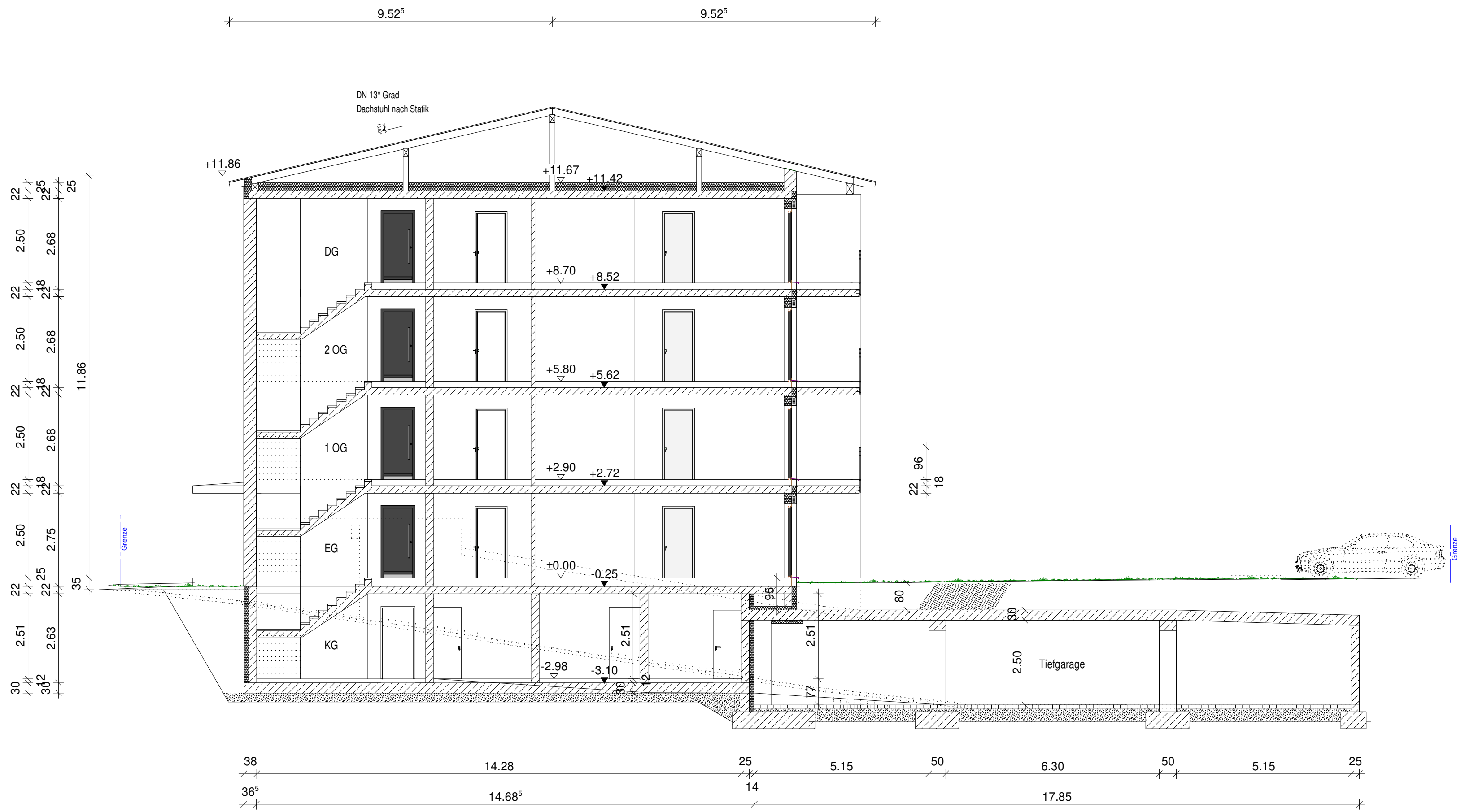
Schnitt D-D Treppenhaus
